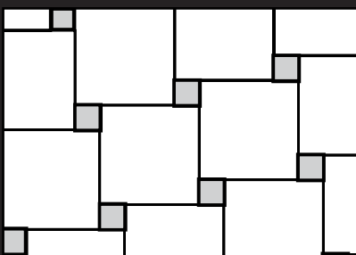
Offsetverlegung mit Schlüsselsteinen offset laying with stone keys pose offset avec cabochons
